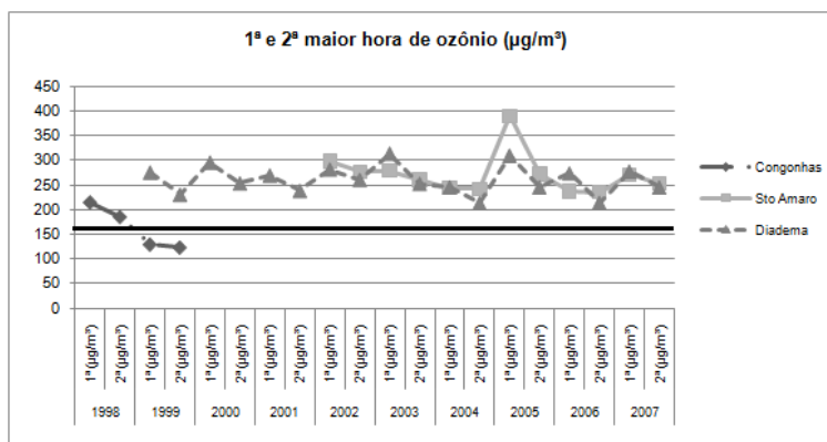
Figura 9 - 1ª e 2ª horas máximas para O 3 nas estações Congonhas, Santo Amaro e Diadema (CETESB).
