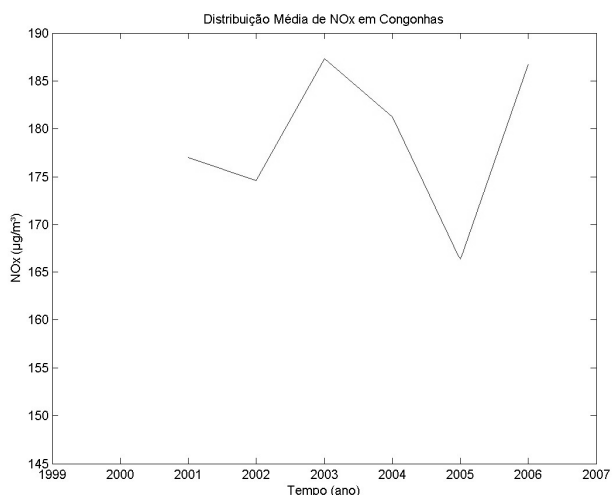
Figura 7 - Distribuição média anual de NO x na estação Congonhas de 1999 a 2007 (CETESB).
